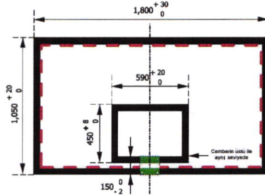
Diyagram 5 - Arkalık işaretleri
