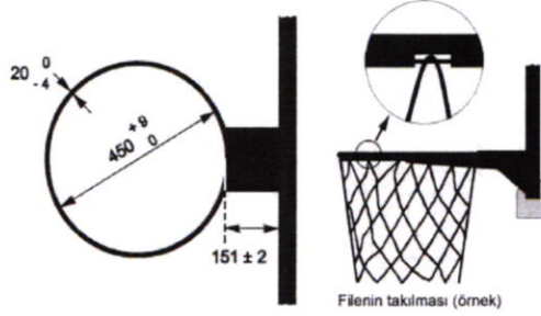
Diyagram 6 - Basket çemberi
