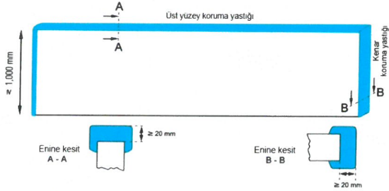
Diyagram12 - Reklam panosu koruma yastığı
