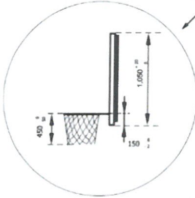
Diyagram 3 - Arkalık ünitesi (şut saati seçenek 1)
