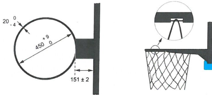
Diagram 6 - Çember boyutları ve File Takılması (örnek)
